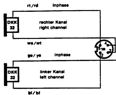
Schaltbild K 141 alte Versionen
