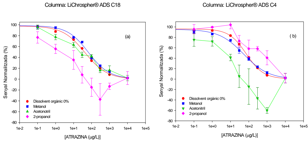
Figura 30 - Corbes de calibratge de l'atrazina amb l'immunosensor en presència de dissolvent orgànic al 40% ((n=4)
