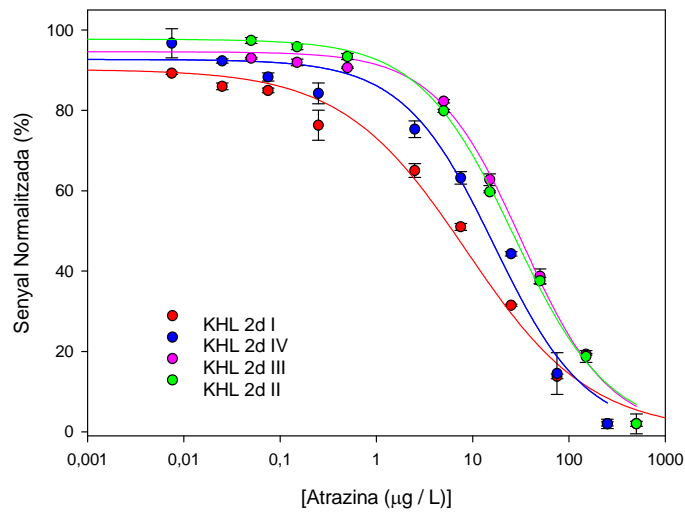
Figura 55 - Corbes de calibratge per l'atrazina amb l'immunosensor H-H utilitzant la bateria d' anticòs i la columna ADS C18 (n=4)
