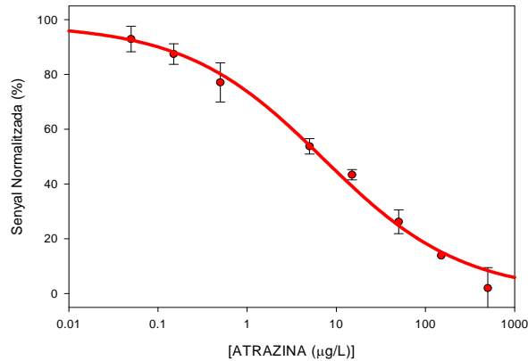
Figura 50 - Corba de calibratge de l' atrazina obtinguda amb l'immunosensor amb etapa prèvia de preconcentració (n=6)
