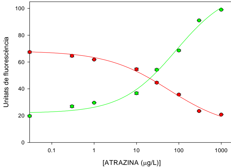
Figura 41 – Corbes de calibratge de l'atrazina amb l'immunosensor obtingudes en format directe (●) i indirecte (●)
