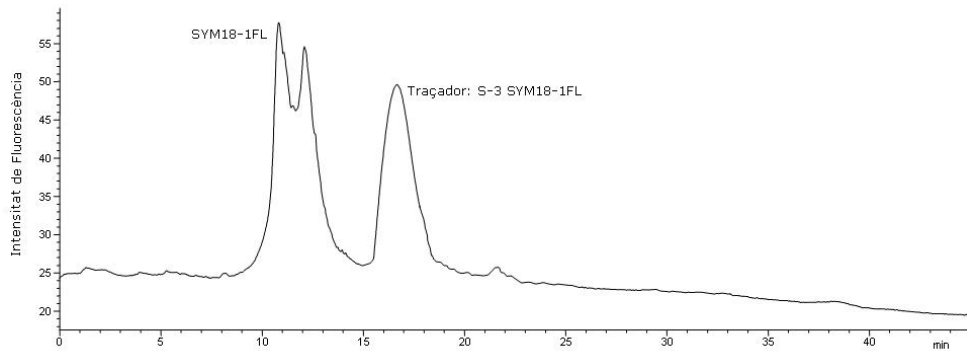
Figura 60 - Cromatograma dels productes de la reacció de conjugació de l'oligonucleòtid SYM 18-1Fl a l'haptè S3
