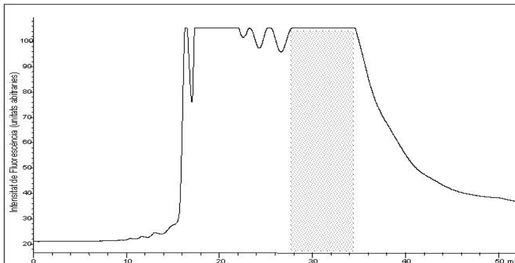
Figura 22 - Cromatograma dels productes de la reacció de conjugació de l'oligonucleòtid SYM18-1FI a l'àcid aspàrtic
