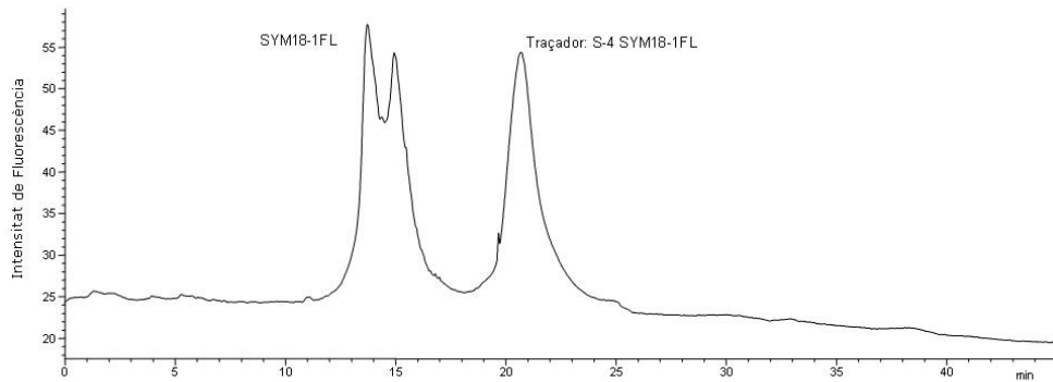
Figura 59 - Cromatograma dels productes de la reacció de conjugació de l'oligonucleòtid SYM18-1Fl a l'haptè S4
