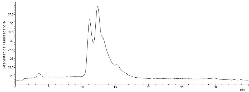
Figura 58 - Cromatograma de l'oligonucleòtid SYM18-1Fl
