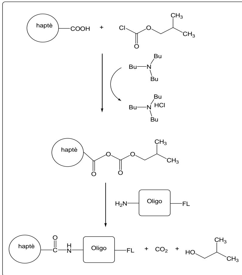
Figura 12 - Protocol d'acoblament d'haptens a oligonucleòtids aminats mitjançant el mètode de l'èster actiu
